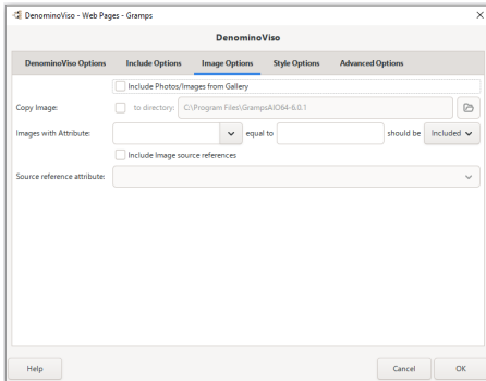
DenominoViso - Web Pages - Addon - "Image Options" tab defaults
