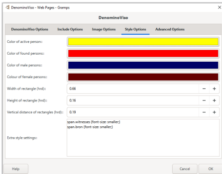
DenominoViso - Web Pages - Addon - "Style Options" tab defaults
